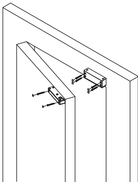
Montage horizontal
